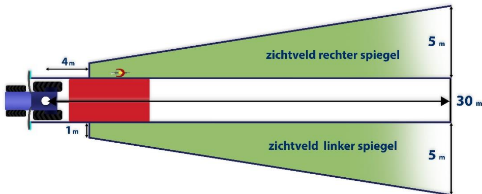
zichtveld tractor
